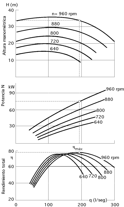
Fig IV.3.- Ensayo completo de una bomba centrífuga a diferente n° de rpm. Curvas, H_m = f(q) ; N = f(q) ; h = f(q)
