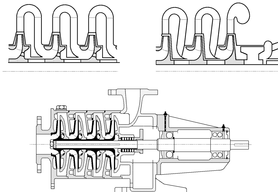
Fig IV.23.- Bomba múltiple constituida por Z rodets iguales acoplados en serie
