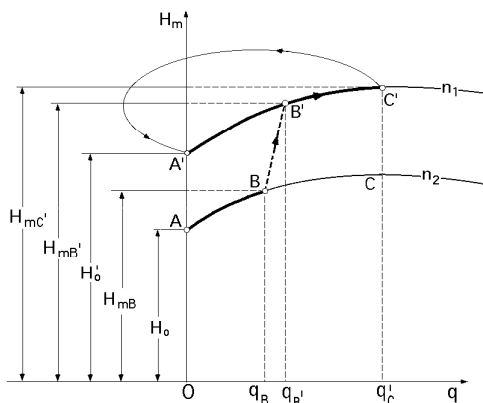
Fig IV.14.- Incremento rápido del caudal proporcionado por la bomba
