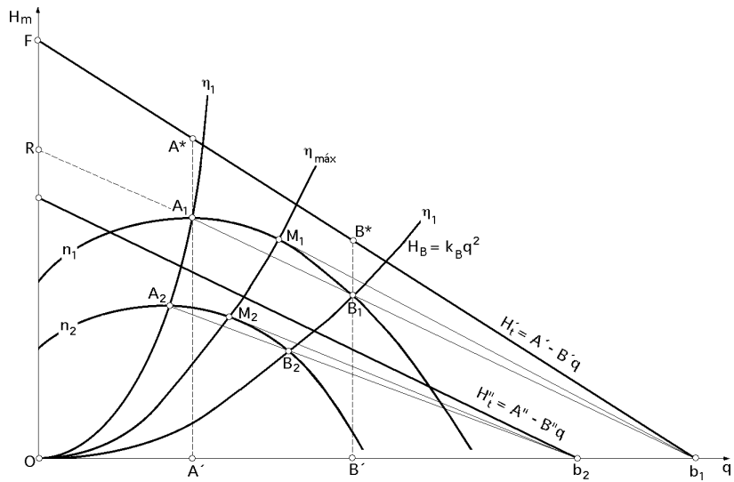
Fig IV.4.- Determinación de los rendimientos en bombas centrífugas
