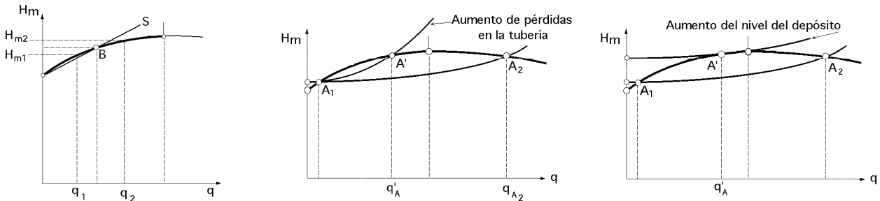
Fig IV.10.- Zona inestable con fluctuaciones
