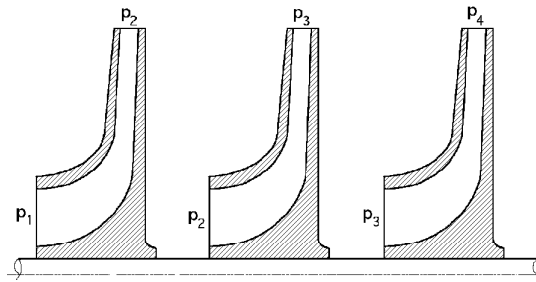
Fig IV.28.- Impulsores idénticos
