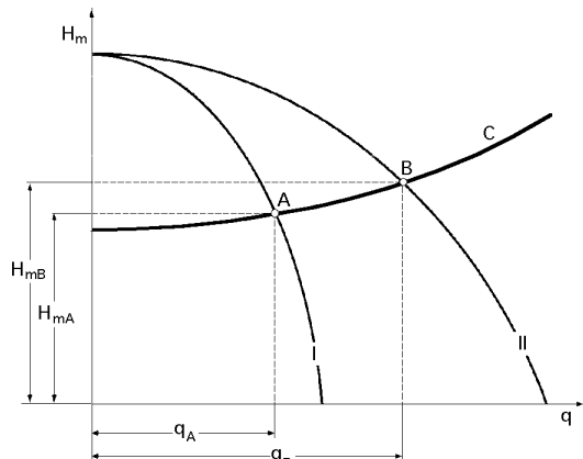
Fig IV.18.- Acoplamiento de bombas idénticas en paralelo
