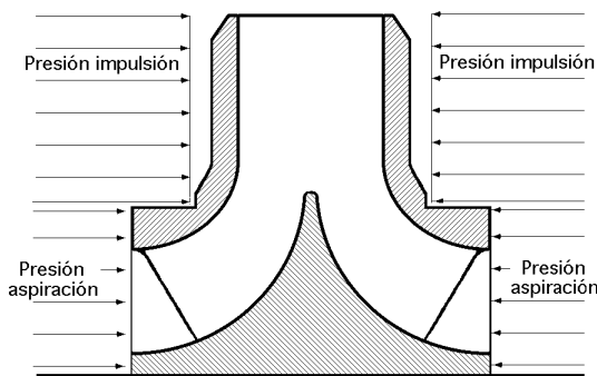
Fig IV.27.- Impulsor de doble aspiración
