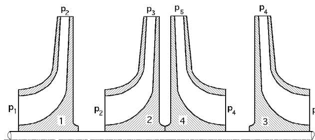
Fig IV.29.- Orden de circulación con varios impulsores
